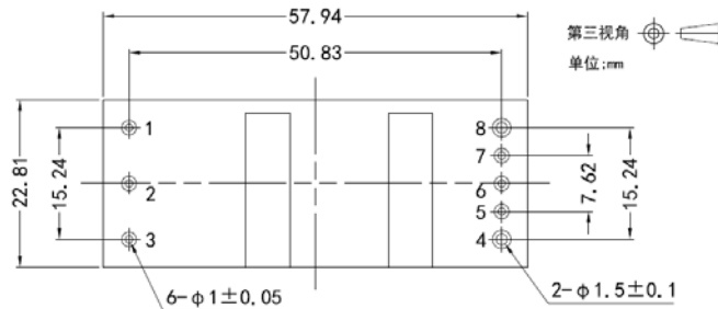
底视图
