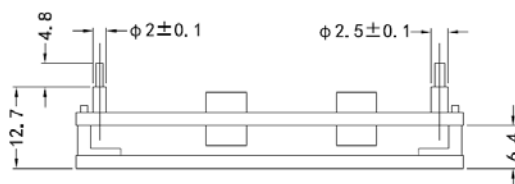
侧视图
