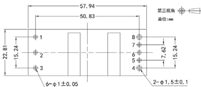
底视图
