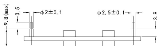
侧视图
